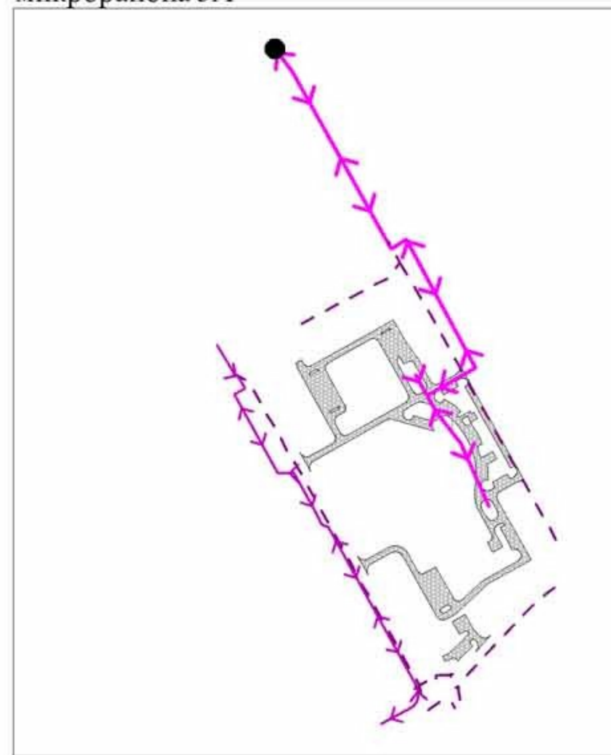
Схема подключения сетей электроснабжения микрорайона 3А
